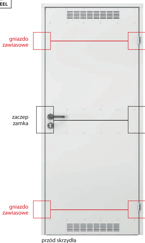
przód skrzydła
