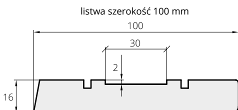
listwa szerokość 100 mm
