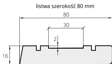
listwa szerokość 80 mm
