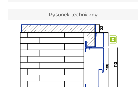
Złożenie ościeżnicy "11" Protect z łącznikiem portalu
