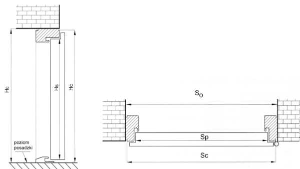
Sposób wymiarowania drzwi z ościeżnicą "11", "12" oraz TERMO i TERMO PRESTIGE
