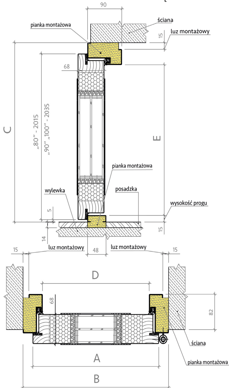
Drzwi z ramką Inox
