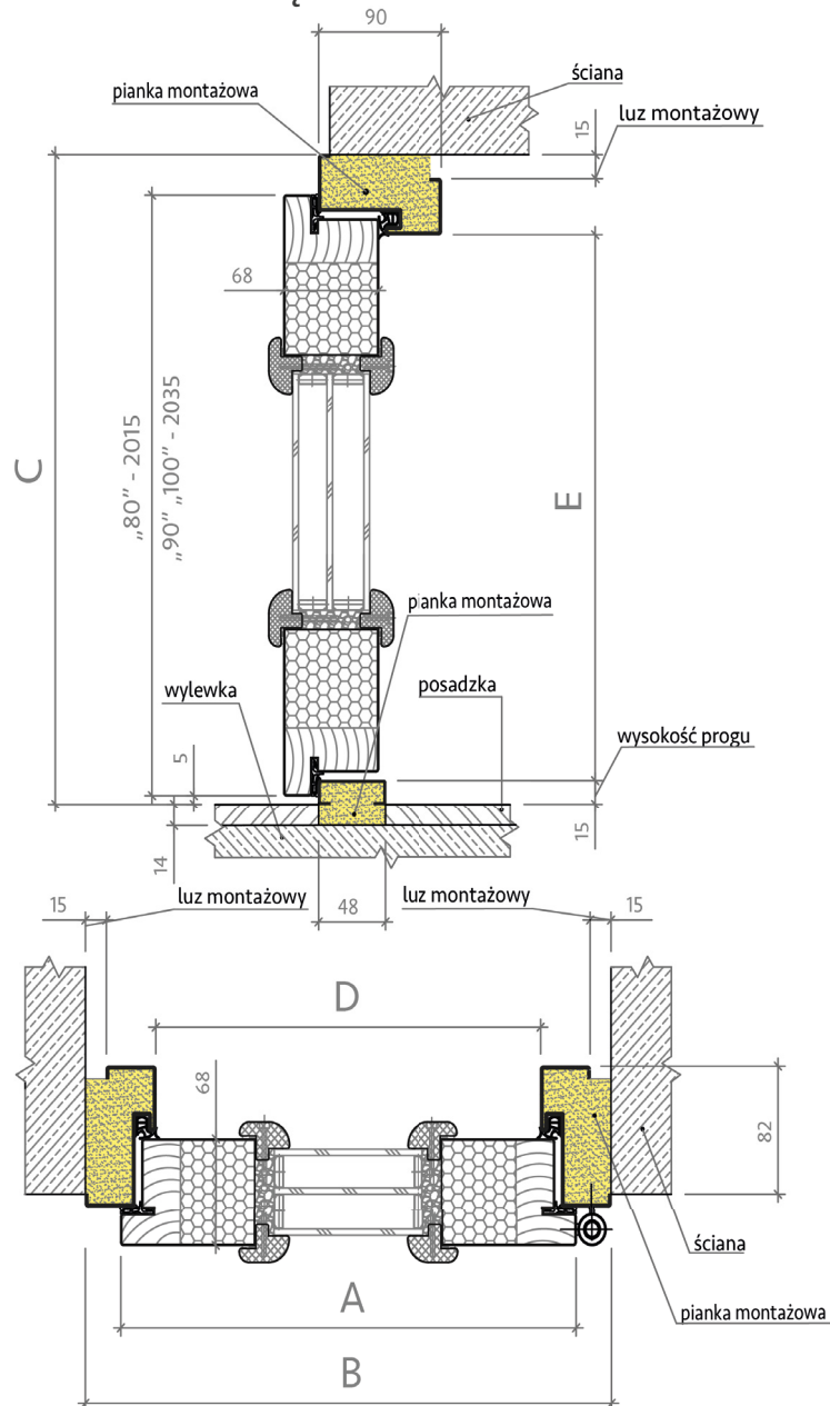
Drzwi z ramką PCV
